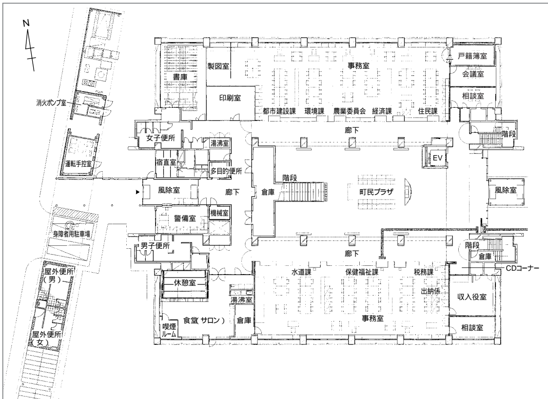
新庁舎1階平面図
