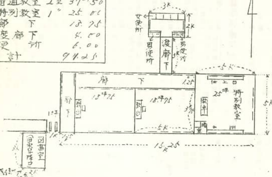
平家3教室(平面図)中学校々舎
