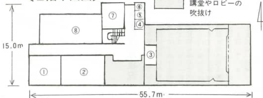
〔2階平面図〕
