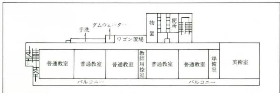
▲ 3階平面図
