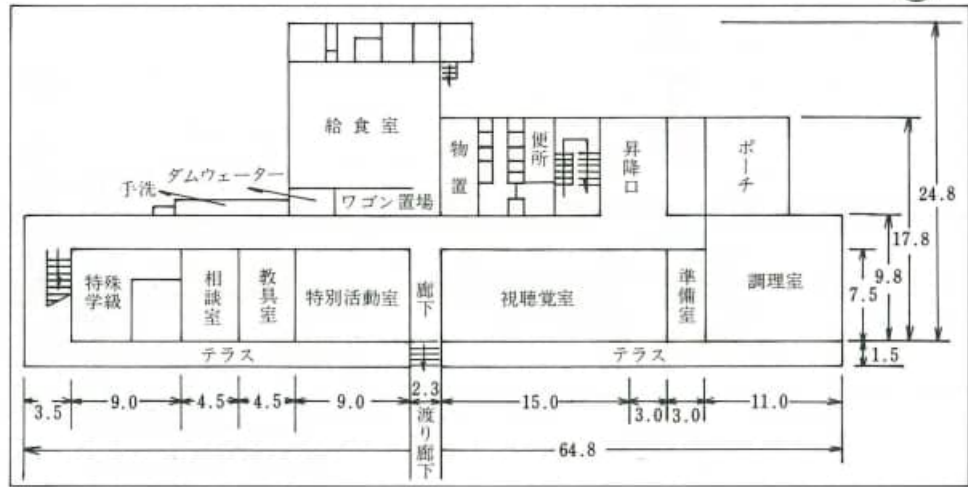
▲ 1階平面図
