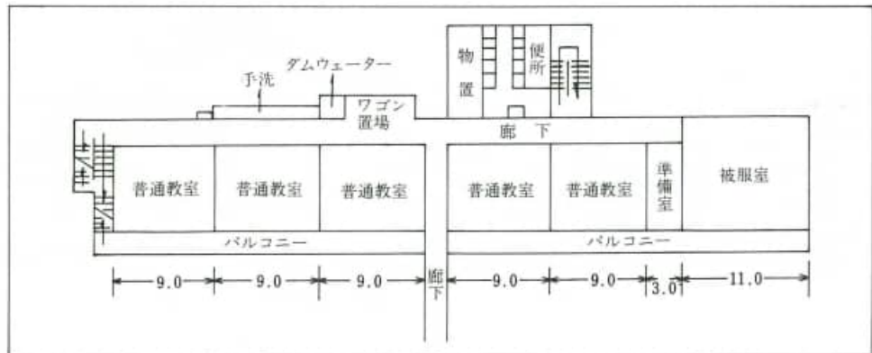
▲ 2階平面図
