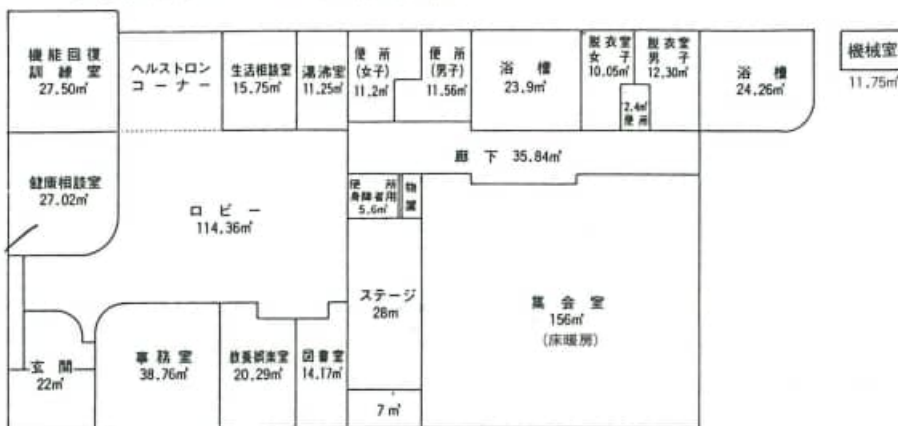
◎老人福祉センター建物平面図
