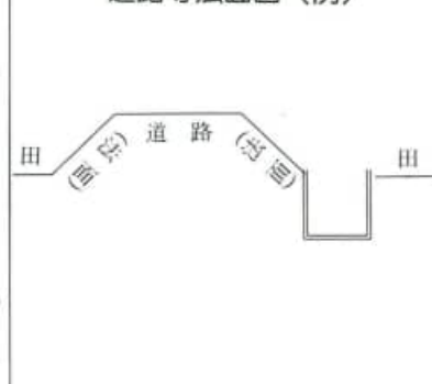
道路等法面図(例)
