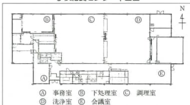
学校給食センター平面図
