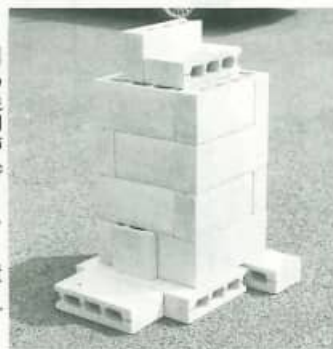
簡易焼却炉(ブロック造り)
