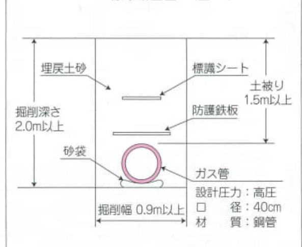
標準断面図 (図-2)
