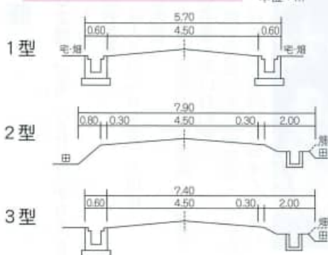
道路改良工事標準横断面図
