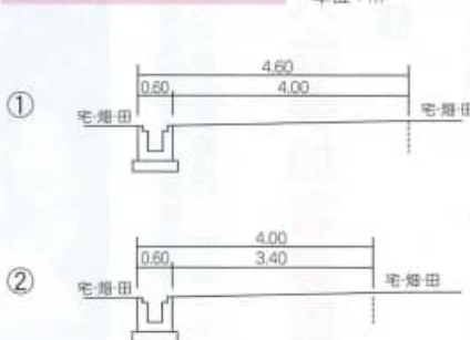
特例道路標準横断面図
