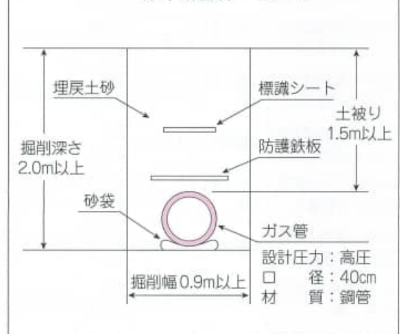
標準断面図 (図-2)
